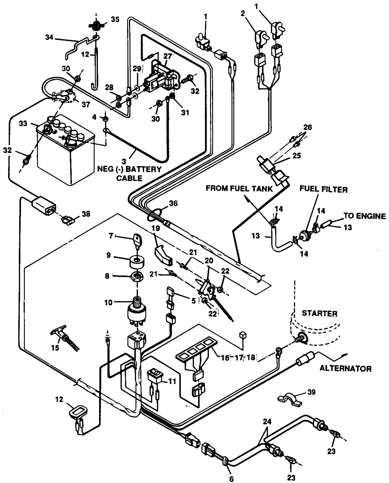
5330577-69 jännitteensäädin
